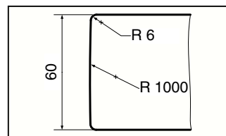
Профиль U-60
