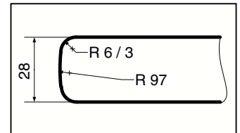
Профиль U-28
