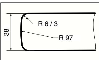
Профиль U-38
