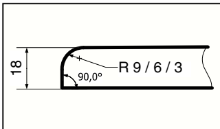
Профиль U-38
