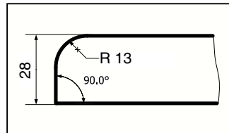
Профиль U-50
